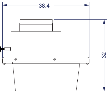
Vista Elevación
